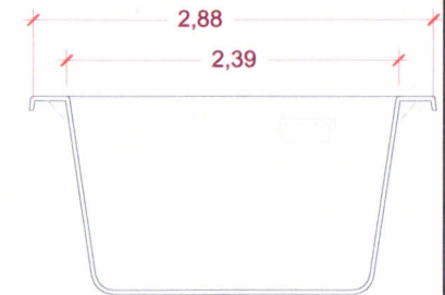
SECCION TRANSVERSAL AA'
