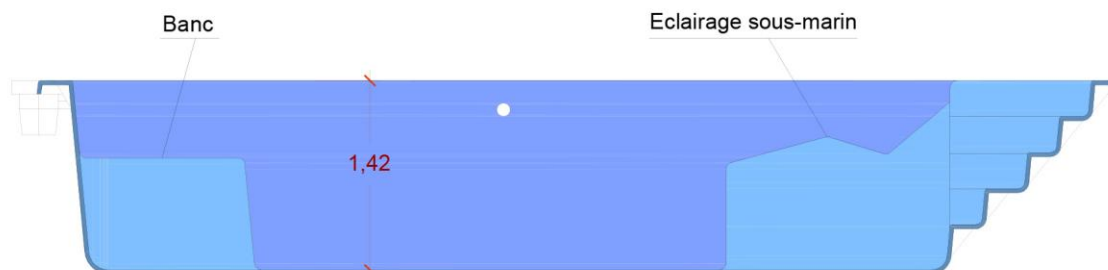
SECTION LONGITUDINALE
