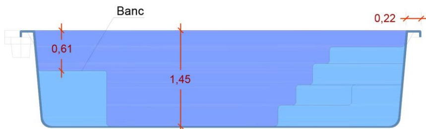
SECTION LONGITUDINALE
