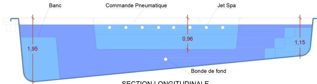
SECTION LONGITUDINALE
