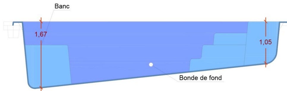
SECTION LONGITUDINALE
